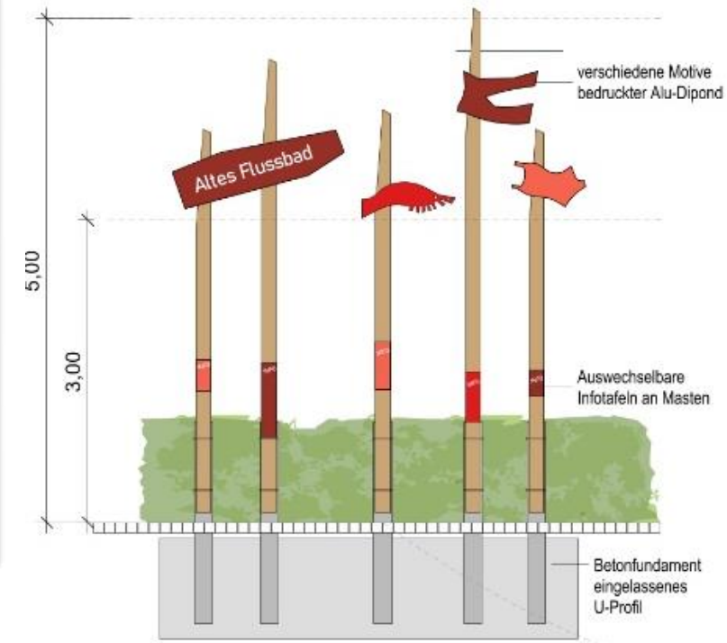
ANSICHT Fahnenmasten mit Infos Parkeingang
